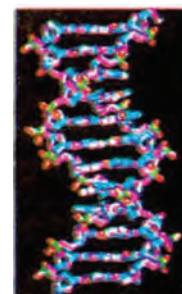
Σχηματική απεικόνιση από υπολογιστή της δομής του μορίου του DNA. Διακρίνονται στη λεπτή έλικα, με γαλάζιο χρώμα τα άτομα του άνθρακα, κόκκινο τα άτομα του οξυγόνου, μωβ τα άτομα του αζώτου, πράσινο τα άτομα του φωσφόρου και λευκό τα άτομα του υδρογόνου
