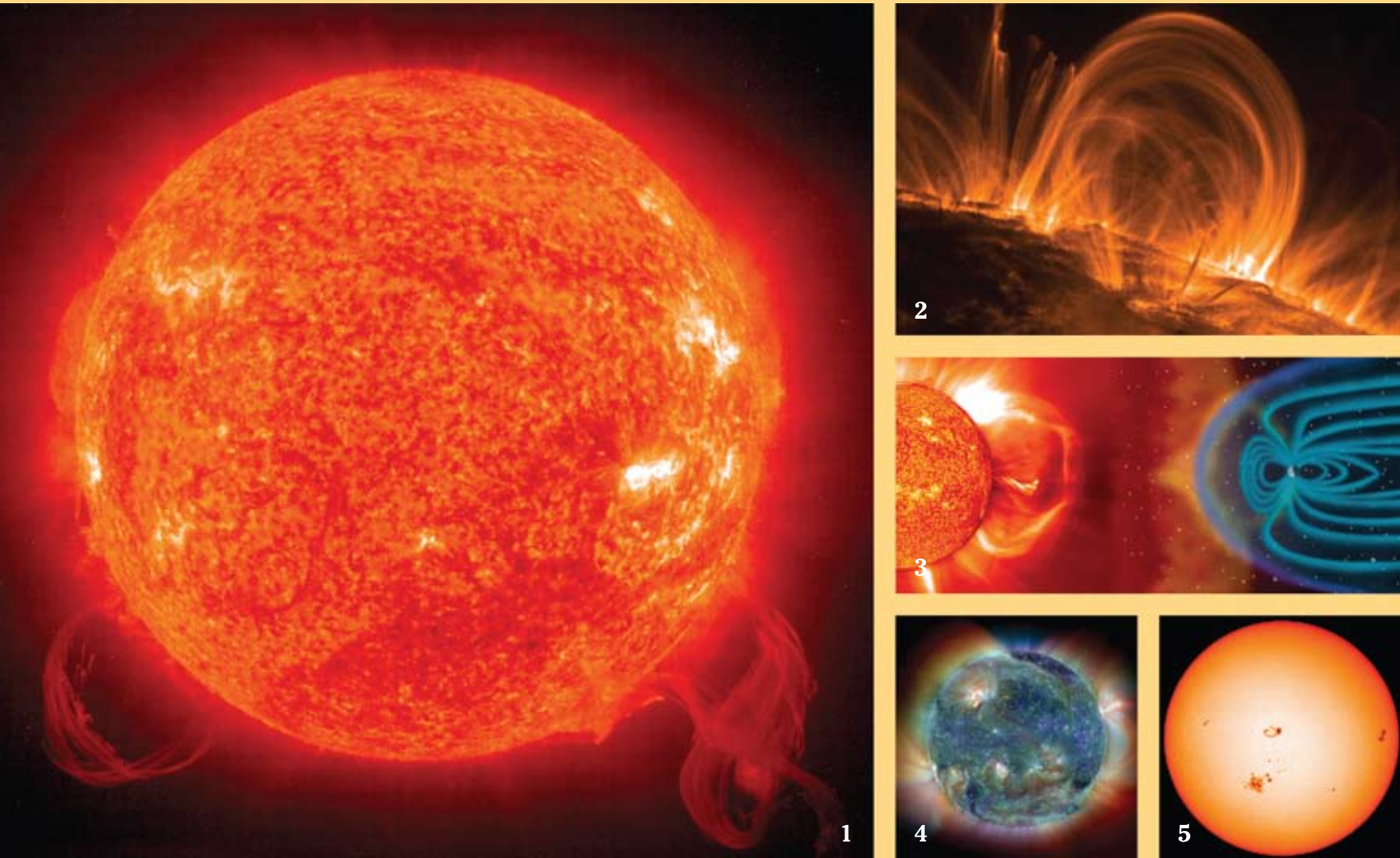
1. Δύο τεράστιες γλώσσες πλάσματος εκτοξεύονται από τη χρωμόσφαιρα του Ηλίου (φωτ. SOHO).
