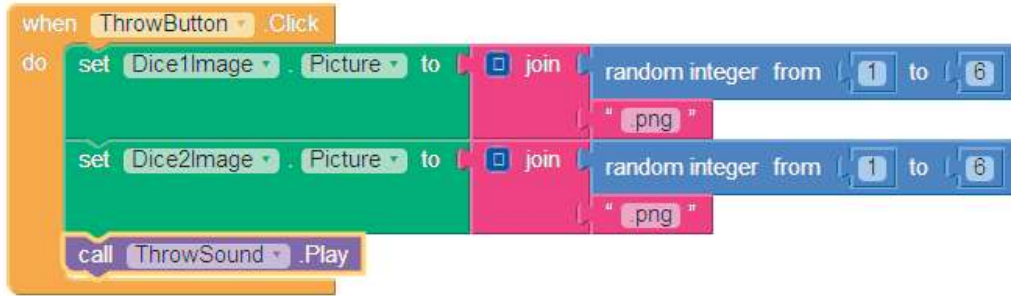
Εικόνα 27 - Τελικό πρόγραμμα Ζάρια
