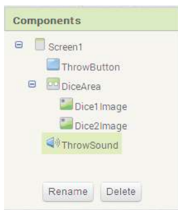
Εικόνα 10 - Μετά την μετονομασία
