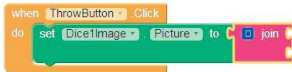
Εικόνα 18 - Μετά την προσθήκη της εντολής join
