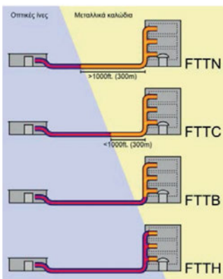
Εικόνα 5.2.α: Τεχνολογίες FttX (πηγή: wikipedia)
