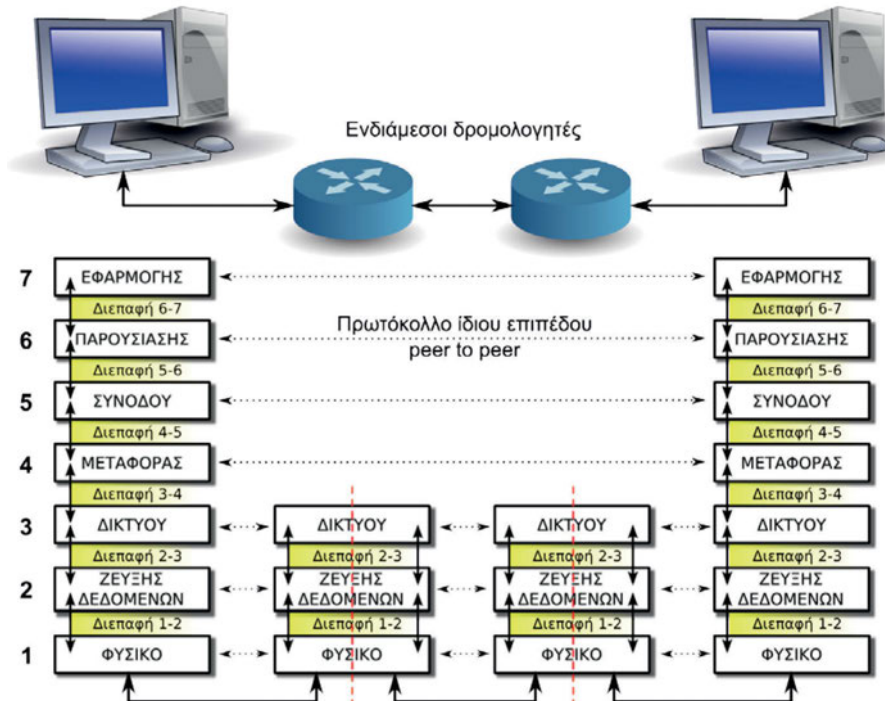
Εικόνα 1.2.1.β: Διαστρωματωμένη αρχιτεκτονική, διεπαφές και ομότιμα επίπεδα
