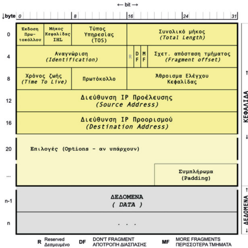
Εικόνα 3.2.α: Το αυτοδύναμο πακέτο IP (IP datagram)
