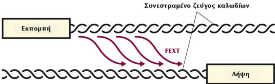
Εικόνα 2.4.1.κ: Παραδιαφωνία FEXT (Far End CrossTalk).
