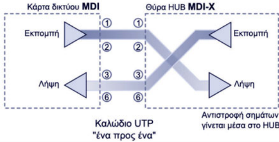
Εικόνα 2.4.3.α:MDI/MDI-X
