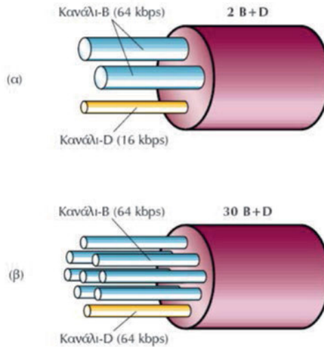
Σχήμα 5.1.3.α. Διεπαφή βασικού ρυθμού BRA (α) και Διεπαφή πρωτεύοντος ρυθμού PRI (β) (Πηγή: Αρβανίτης, Κ., Κολυβάς, Γ., & Ούτσιος, Σ. (2001). Τεχνολογία Δικτύων Επικοινωνιών)
