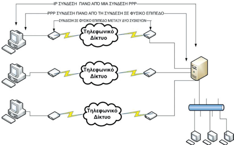
Εικόνα 2.7.α: Εγκατάσταση σύνδεσης με πρωτόκολλο Σύνδεσης Σημείου προς Σημείο (PPP)
