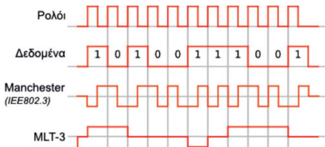
Εικόνα 2.4.1.κζ: Κωδικοποίηση Manchester, MLT-3
