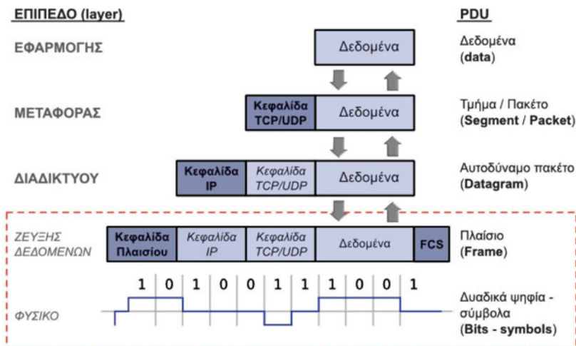
Εικόνα 1.3.α: Ενθυλάκωση
