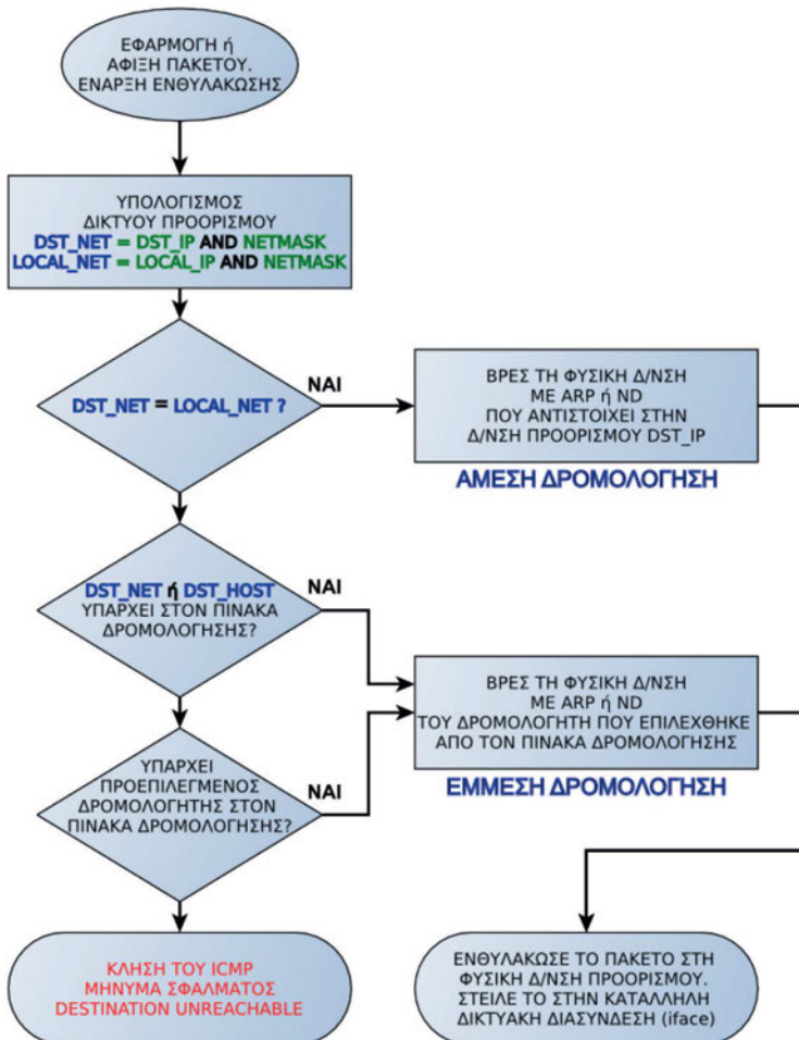
Σχήμα 3.6.1.α: Διαδικασία δρομολόγησης αυτοδύναμου πακέτου
