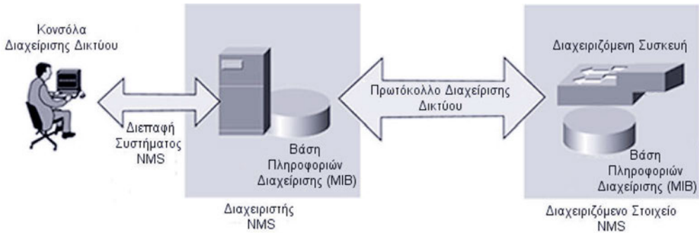
Εικόνα 7.1.α: Βασική δομή Συστήματος Διαχείρισης Δικτυού (NMS)
