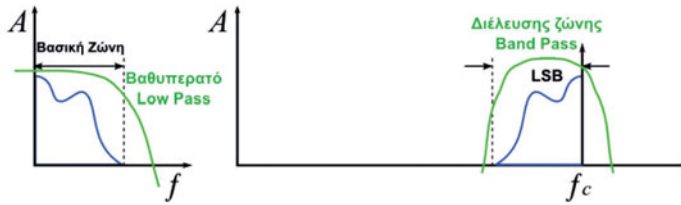
Σχήμα 2.3.α: Βασική ζώνη (Low Pass).
