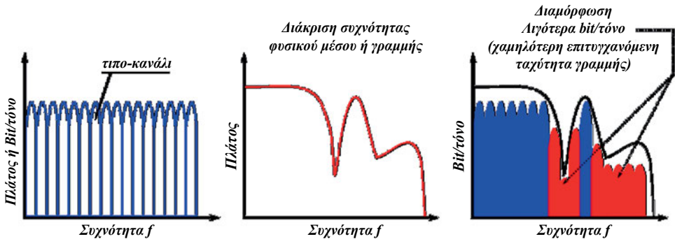
Εικόνα Π.3.α: Διαμόρφωση Διακριτής Πολυτονίας (DMT)
