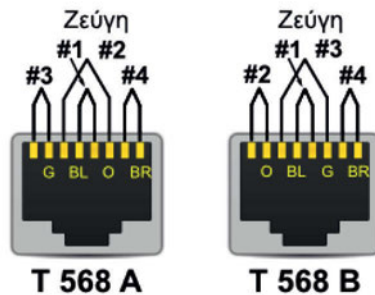
Εικόνα 2.4.1.α: Συρμάτωση
