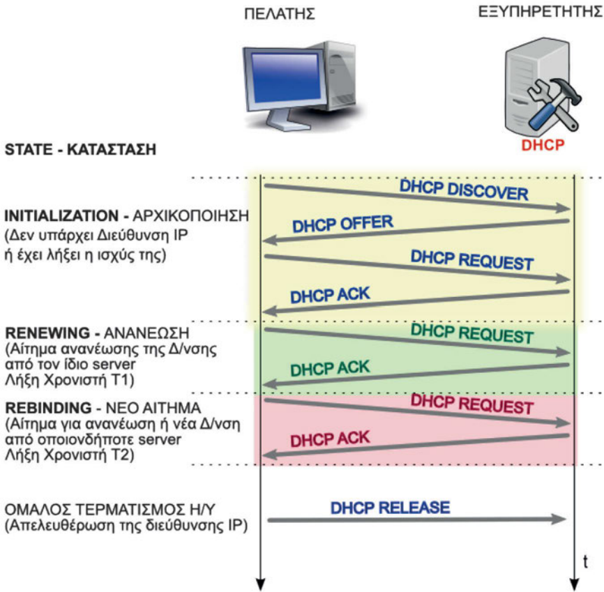
Εικόνα 3.2.2.α: Λειτουργία DHCP
