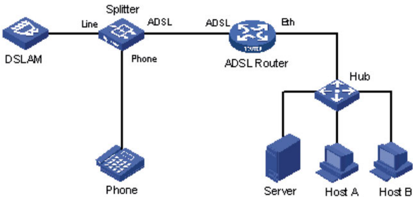
Σχήμα 5.1.4.2.α. Τοπολογία ADSL
