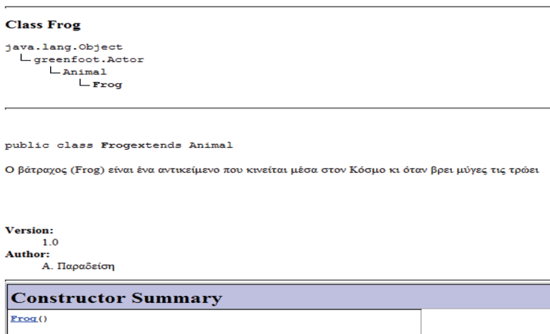
Εικόνα 2.5.6 Τεκμηρίωση της κλάσης Frog
