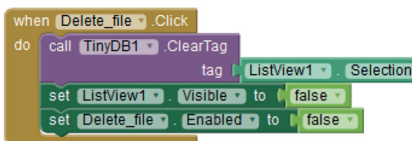
Εικόνα 19.3.1. Διαγραφή από τη βάση.
