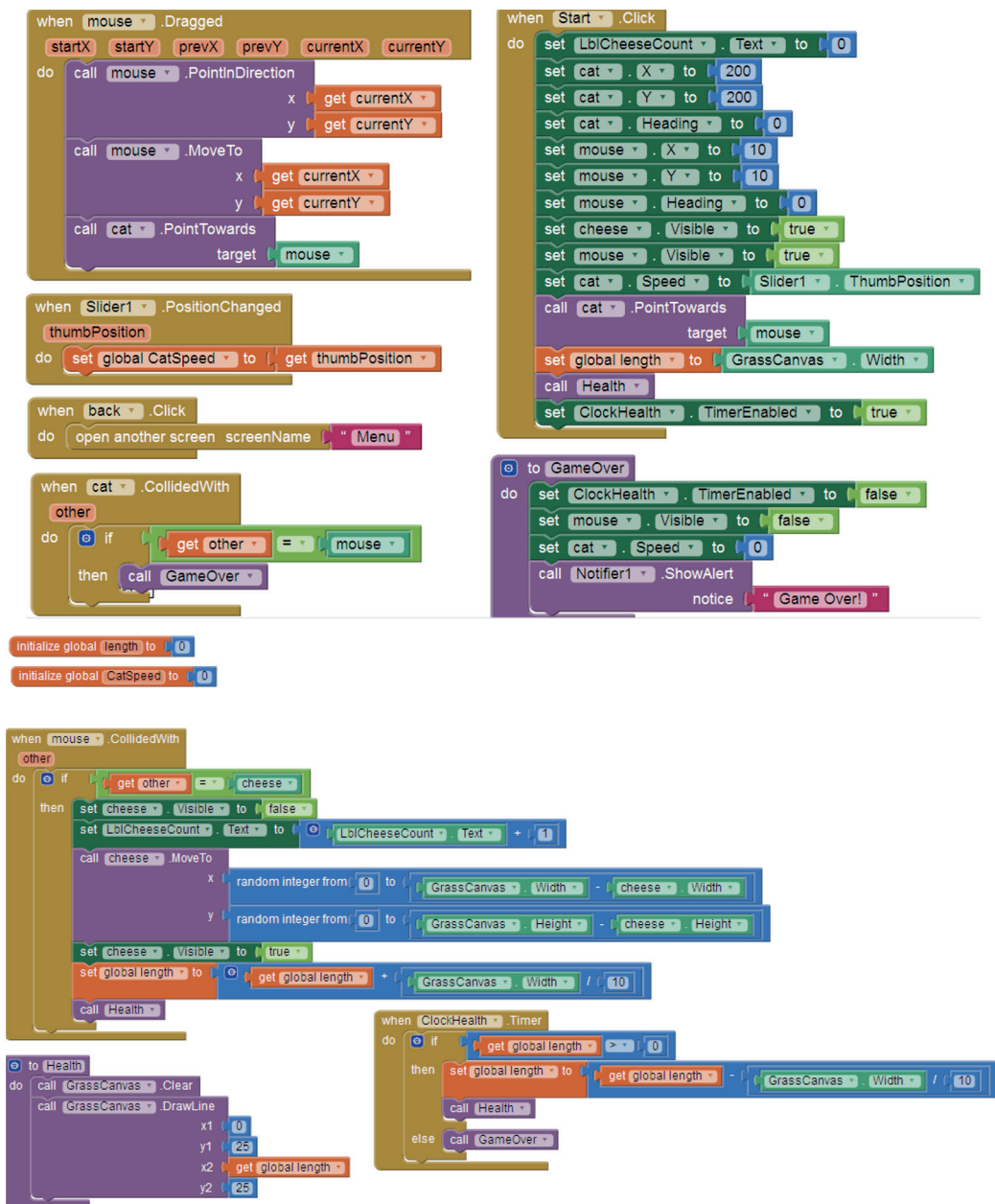
Εικόνα 15.3.1. Το πρόγραμμα για την οδόνη Chase.
