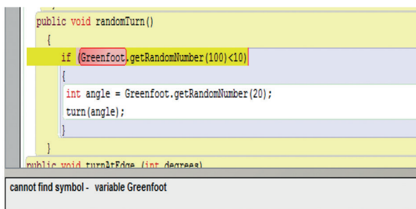
Εικόνα 3.8.1 Μήνυμα λάθους σε κλήση μεθόδου άλλης κλάσης
